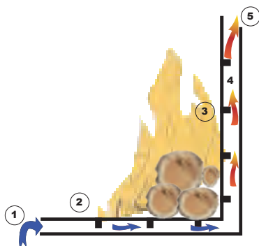
Récupérateur de chaleur à air encastrable
